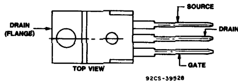
92CS-39528 JEDEC TO-220AB
